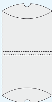
CAIXA PASTEL (com picote) LAR. 15 X COMP. 25 X LAT. 4,6
