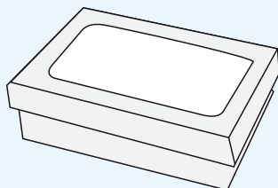
CAIXA C/ VISOR - 01 LARG. 15,5 X COMP. 23,5 X ALT. 6,2
