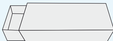
CAIXA P LARG. 17,7 X COMP. 7,5 X ALT. 4,0
